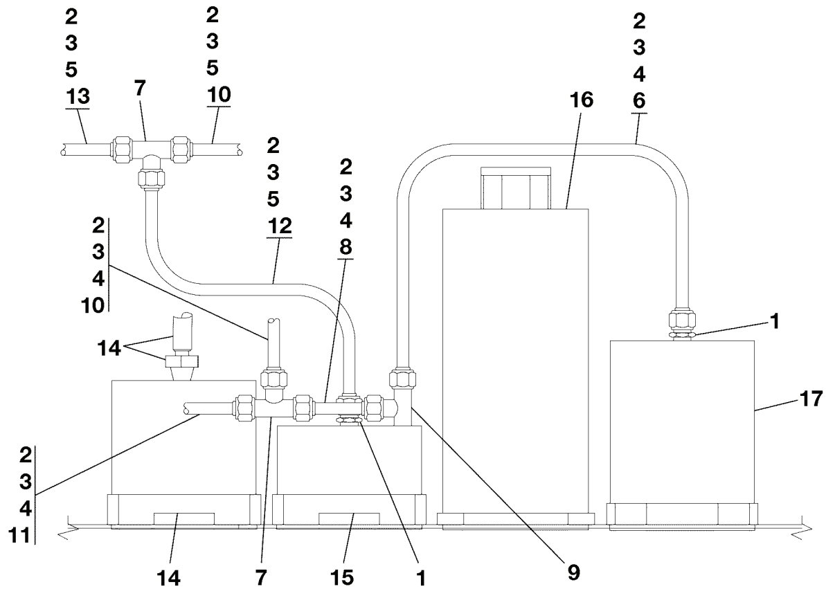
VIEW A-A
