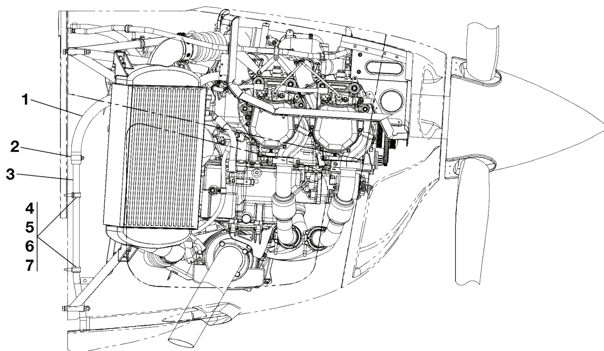
VIEW A-A
