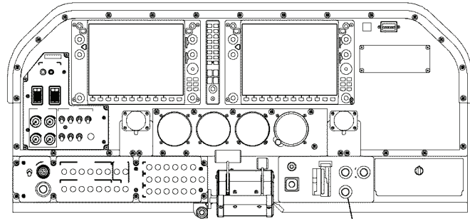
VIEW A-A
