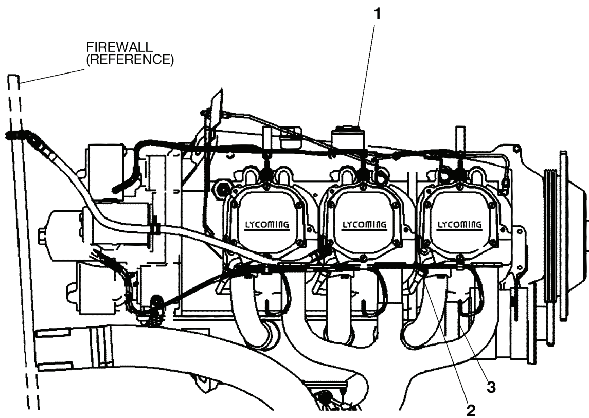
VIEW A-A
